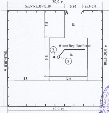
План огорожі М 1:500
