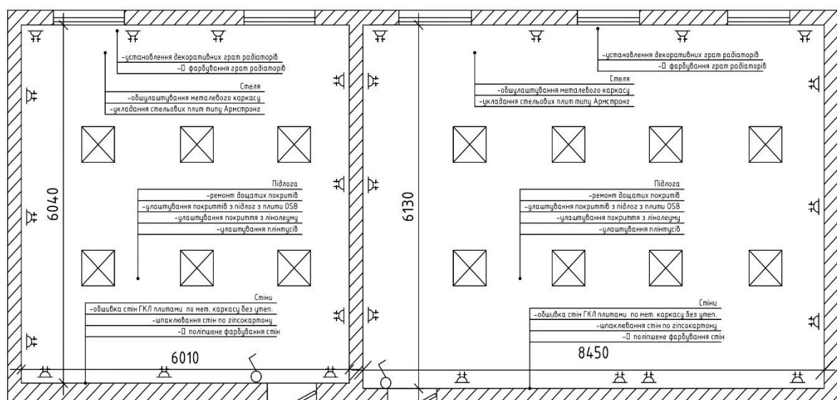
Схема виконання робіт Поточний ремонт приміщень громадського простору, по провулку Шкільному, 8 селищі Краснокутськ, Богодухівського району, Харківської області
